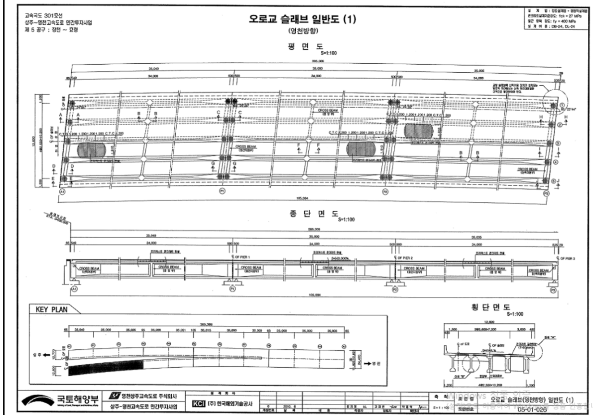
【그림 9.1.4】 슬래브 일반도
