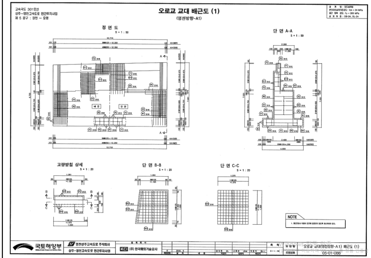
【그림 9.1.9】 교대 배근도
